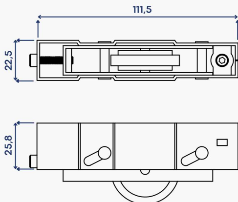
ESCALA 1:2
