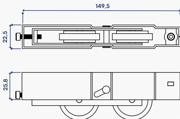
ESCALA 1:2
