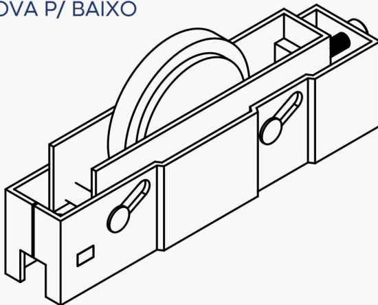
DIMENSÕES (mm)
