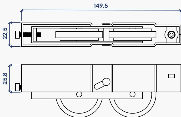
DIMENSÕES (mm)
