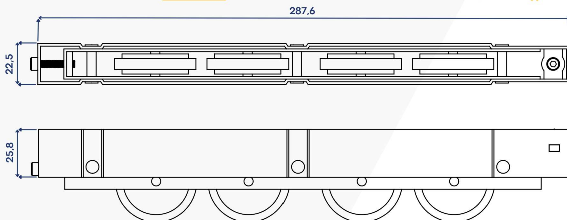
ESCALA 1:2
