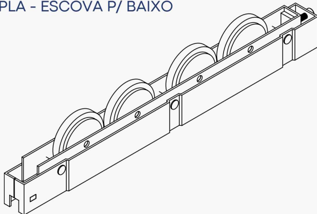
DIMENSÕES (mm)
