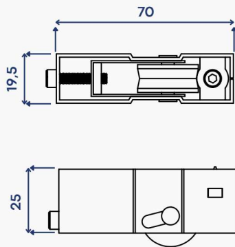
DIMENSÕES (mm)
