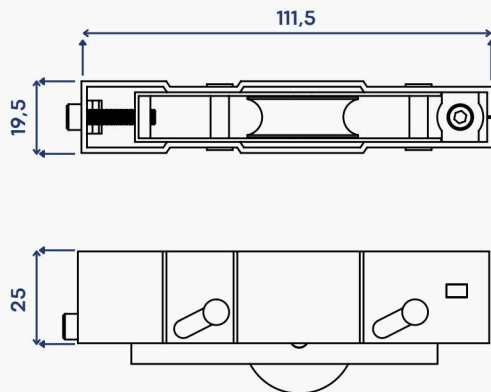
DIMENSÕES (mm)
