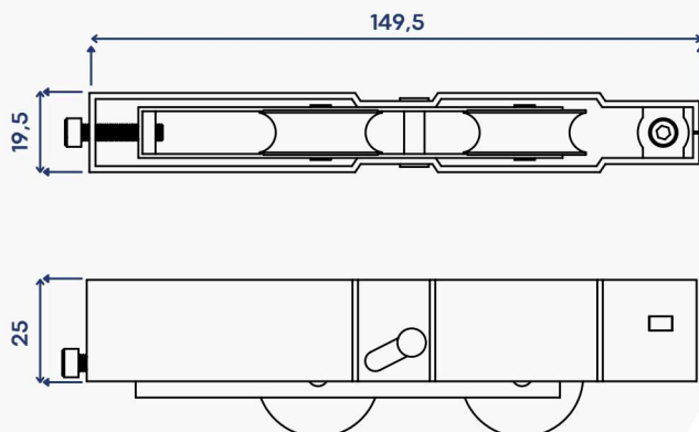
DIMENSÕES (mm)
