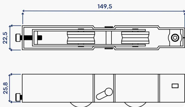
DIMENSÕES (mm)
