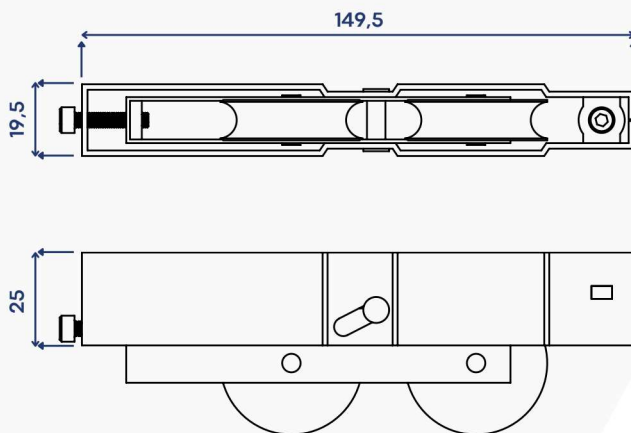
ESCALA 1:2
