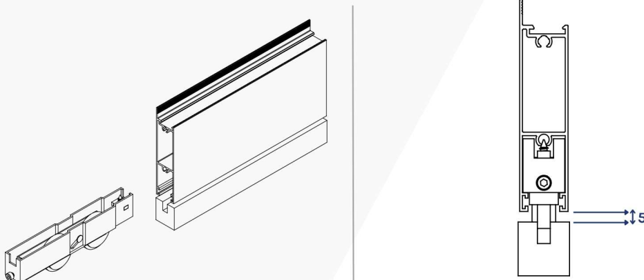
DETALHE DE APLICAÇÃO (sem escala)
