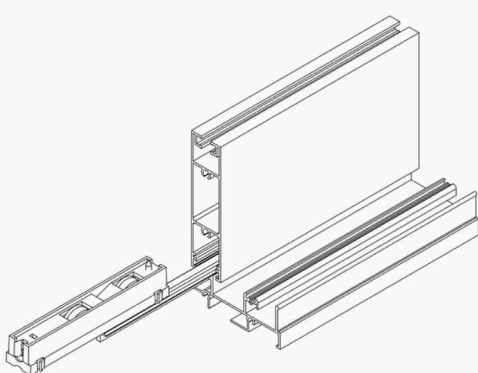
DETALHE DE APLICAÇÃO (sem escala)
