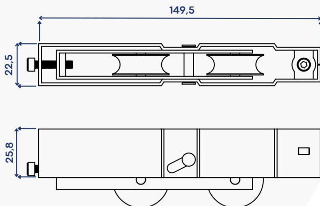
DIMENSÕES (mm)
