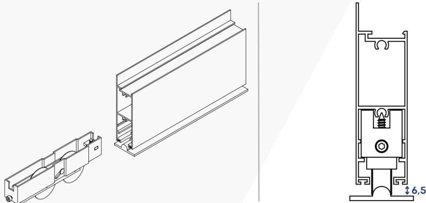
DETALHE DE APLICAÇÃO (sem escala)
